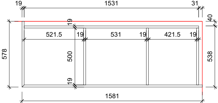
B-B Sockelplan
